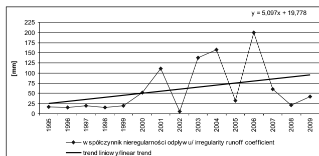
Ryc. 8. Współczynnik nieregularności odpływu dla Bystrzanki w latach 1995–2009 Fig. 8. Irregular runoff coefficient for Bystrzanka stream in period 1995–2009
